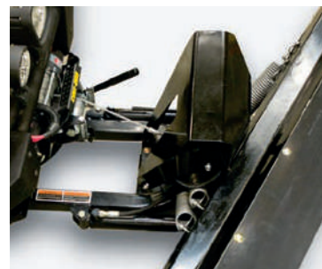
Электрогидравлический блок
